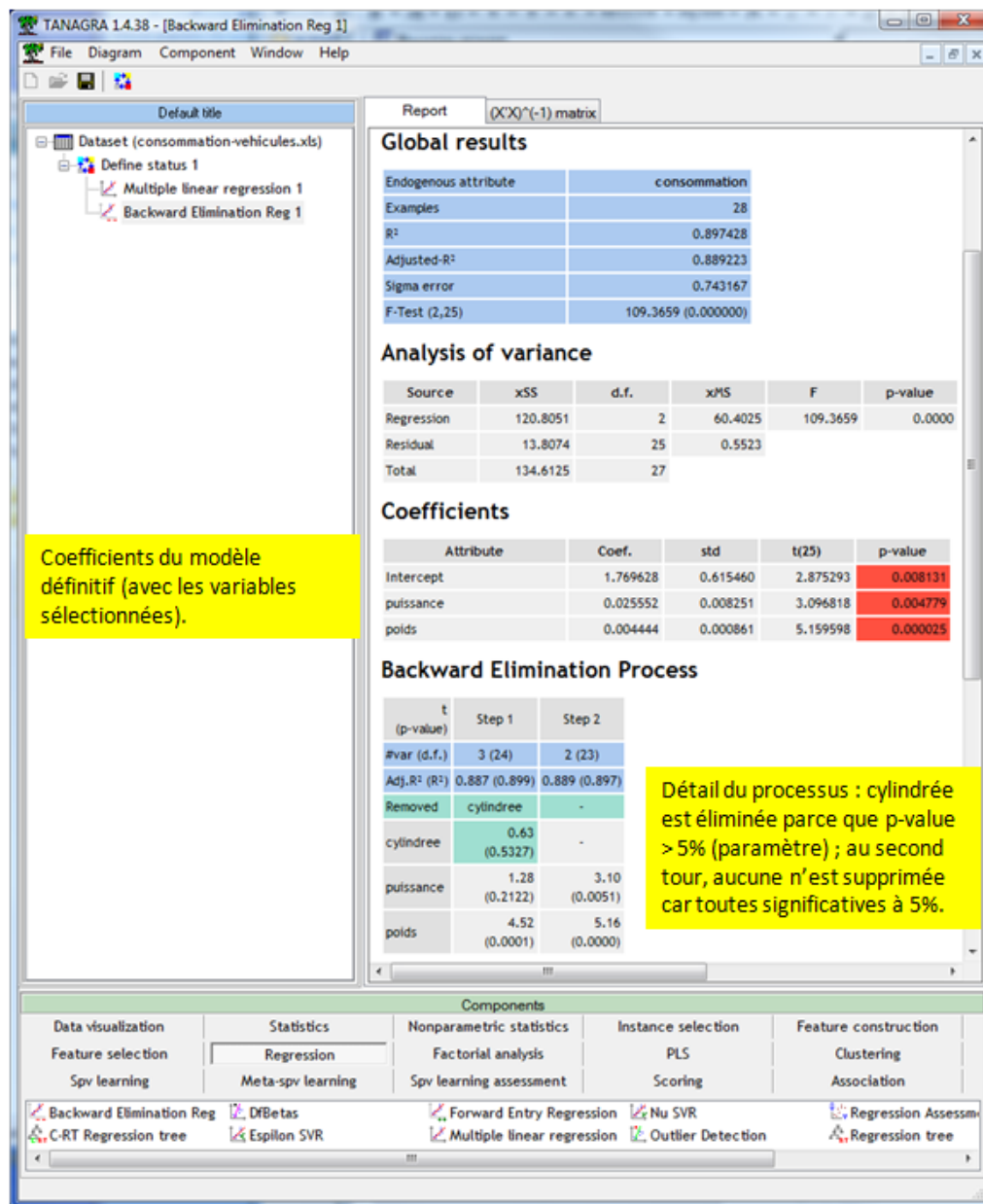
Fig. 15.4. Utilisation du composant "Backward Elimination Reg" dans Tanagra - Consommation des véhicules
