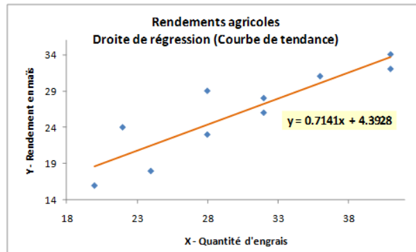
Fig. 1.5. Droite de régression - "Rendements agricoles"
